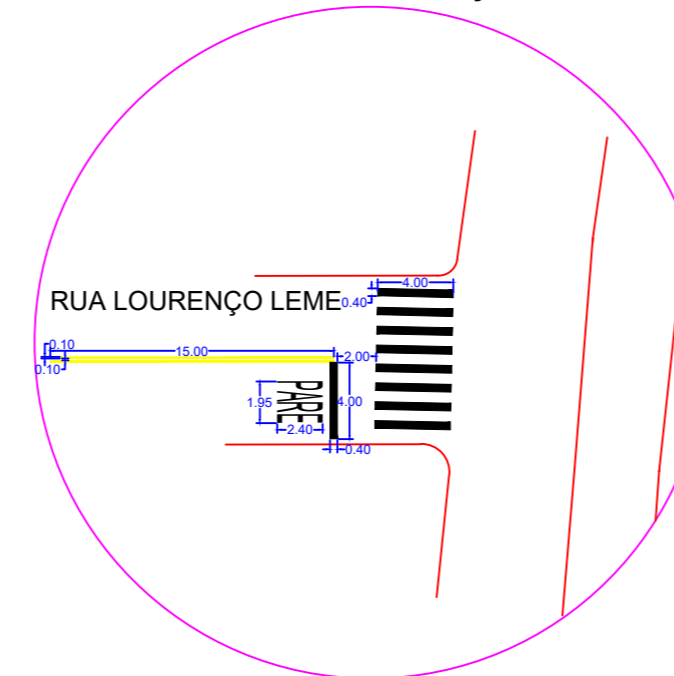
CRUZAMENTO TIPO 05 Pintura demarcação
