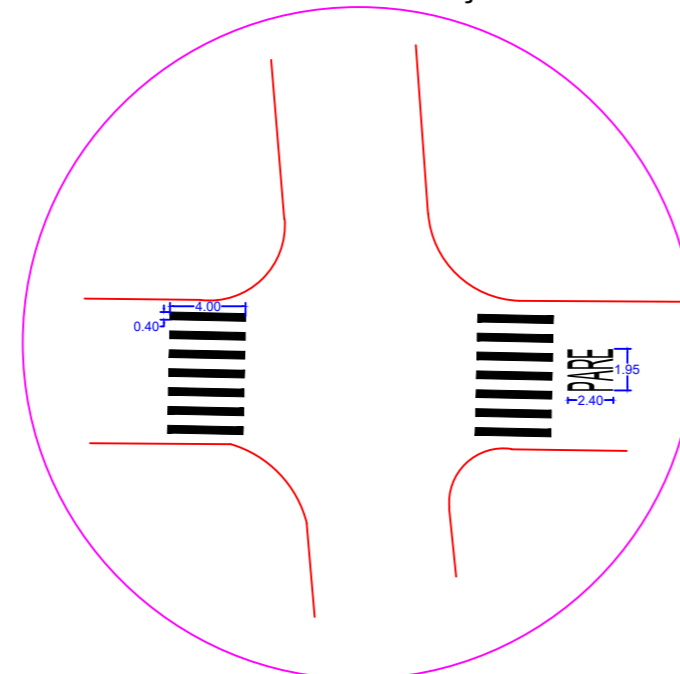
CRUZAMENTO TIPO 07 Pintura demarcação
