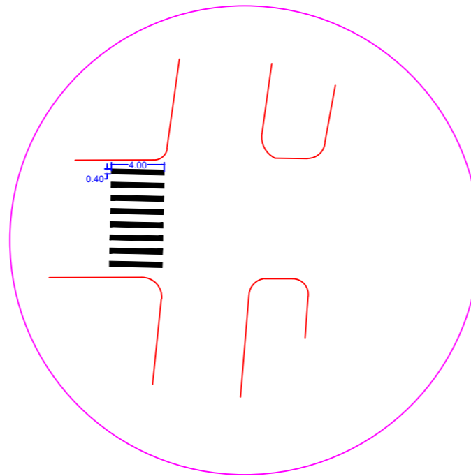
CRUZAMENTO TIPO 02 Pintura demarcação
