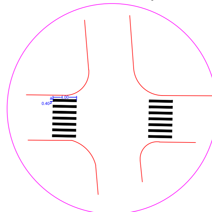
CRUZAMENTO TIPO 06 Pintura demarcação
