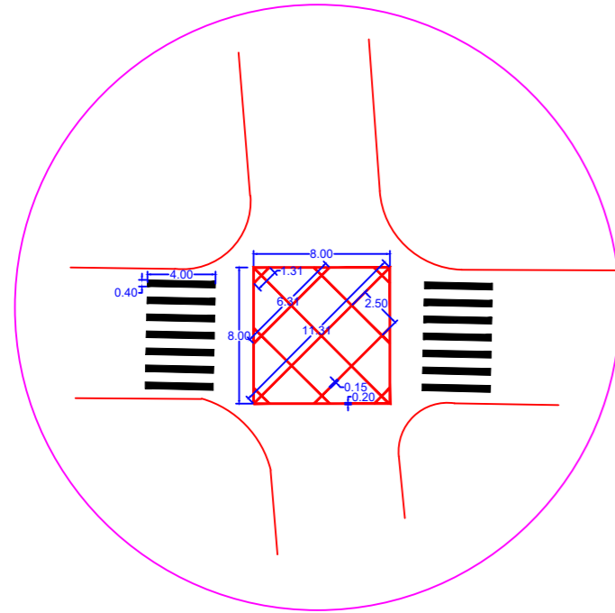
CRUZAMENTO TIPO 01 Pintura demarcação
