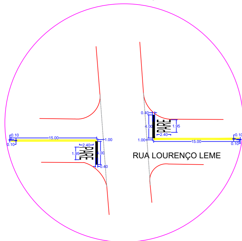
CRUZAMENTO TIPO 04 Pintura demarcação
