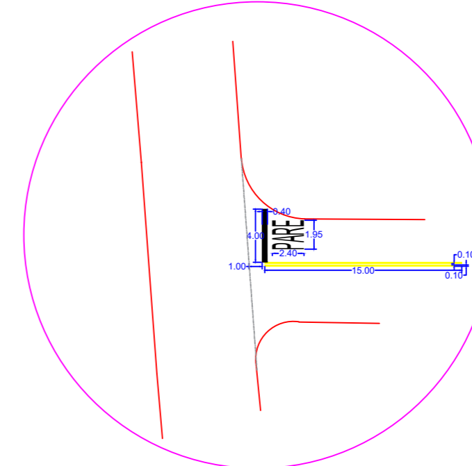
CRUZAMENTO TIPO 03 Pintura demarcação
