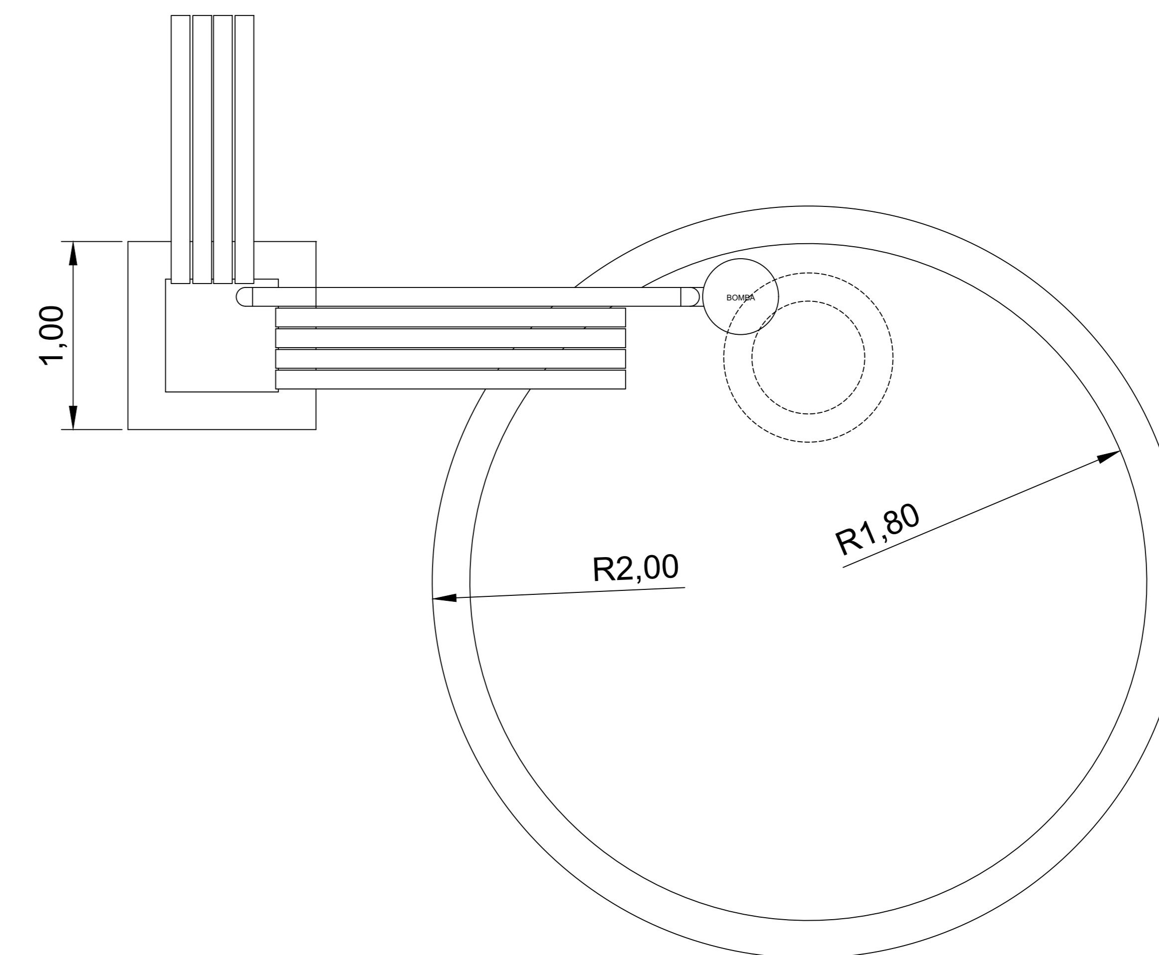
RESERVATÓRIO DE ÁGUA DE CHUVA - PLANTA
