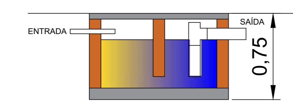
CAIXA DE GORDURA - CORTE
