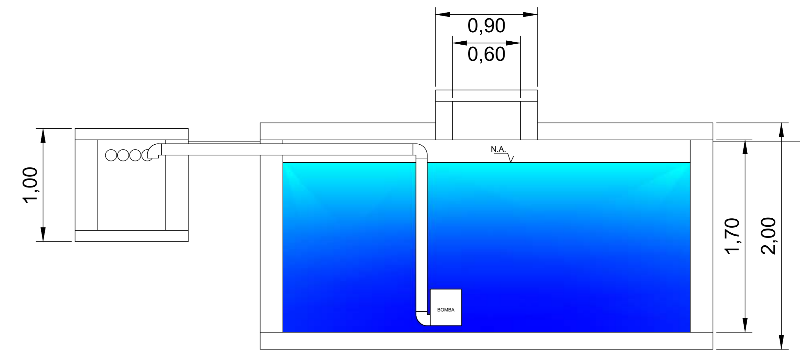
BOMBA DE DRENAGEM - CORTE
