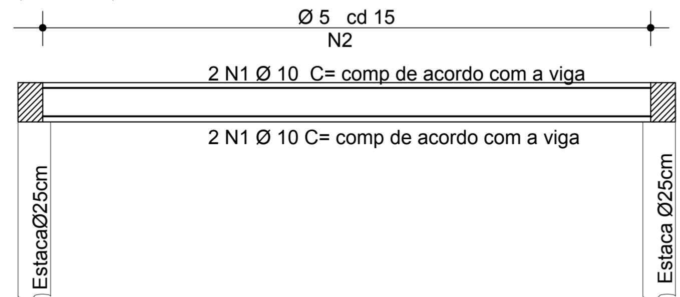
DETALHE TÍPICO DAS VIGAS BALDRAMES 30X30CM (SEM ESCALA)
