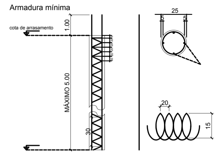
DETALHE TÍPICO DAS ESTACAS Ø 25cm e prof=5,00m (SEM ESCALA)
