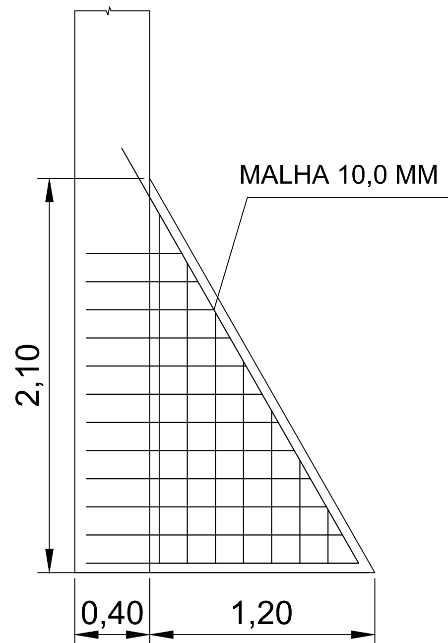
ARMADURA CONTRAFORTES
