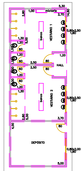
VESTIÁRIO / DEPÓSITO ESCALA 1:200
