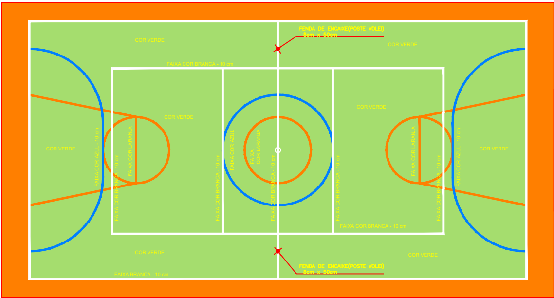
PINTURA QUADRA - ÁREA 480m² ESCALA 1:200
