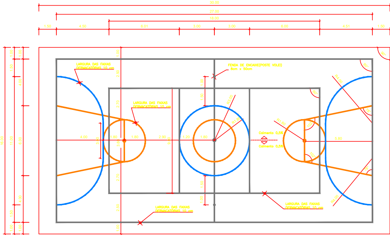
MEDIDAS QUADRA ESCALA 1:200
