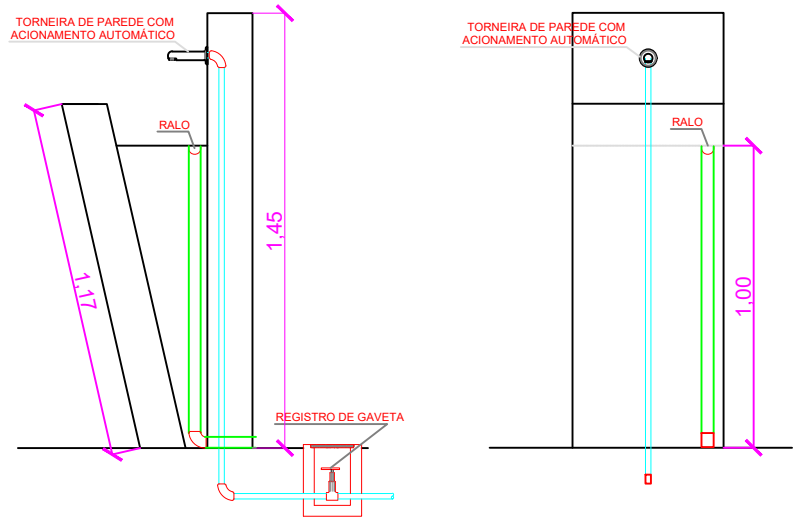
DETALHE - BEBEDOURO ESCALA 1:25
