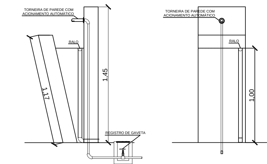
DETALHE — BEBEDOURO ESCALA 1:25
