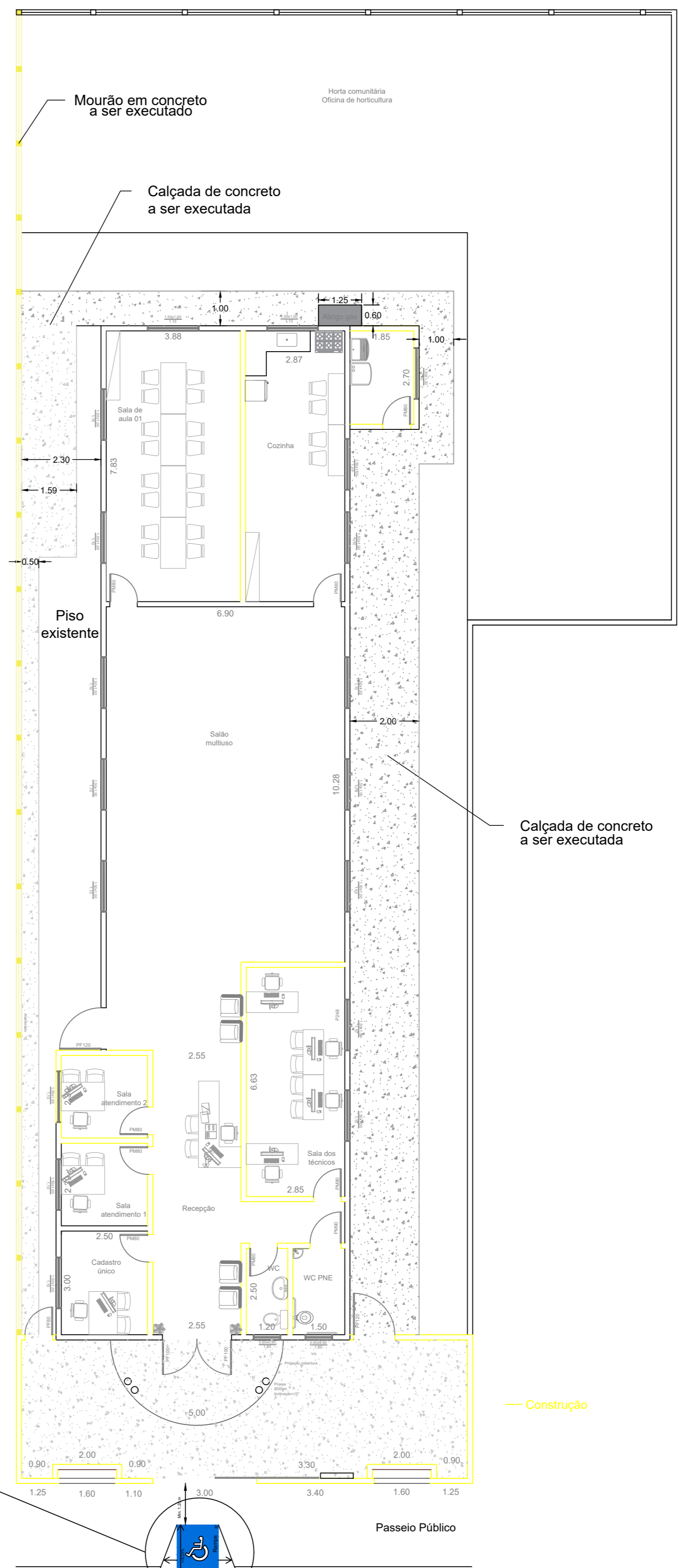
Planta baixa - Situação final Escala 1:100
