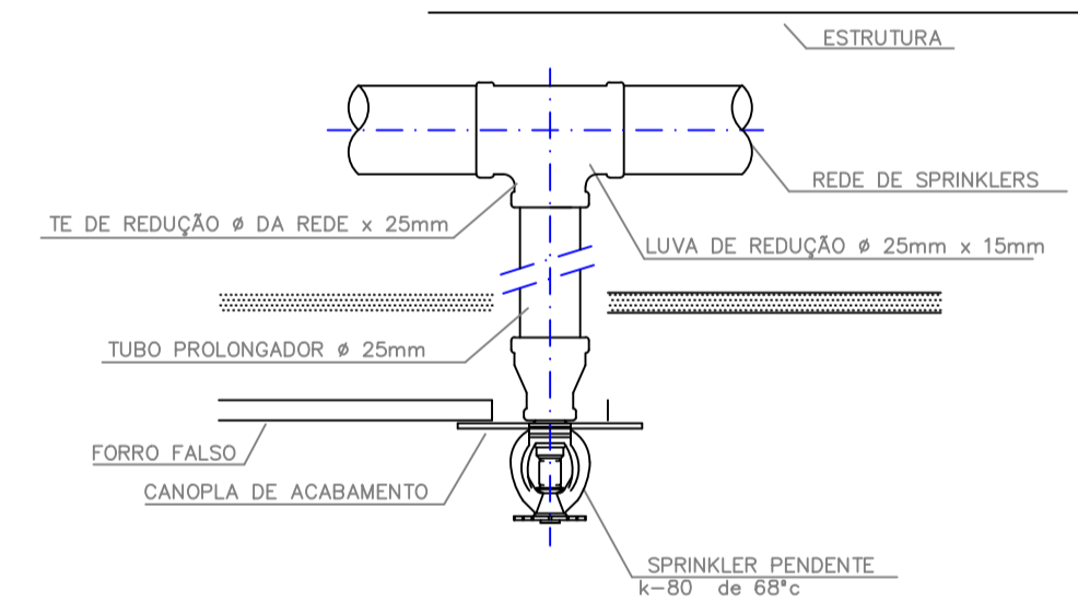
DET. DE INSTALAÇÃO DE SPRINKLER PENDENTE EM AREA COM FORRO FALSO – FP018 SEM ESCALA
