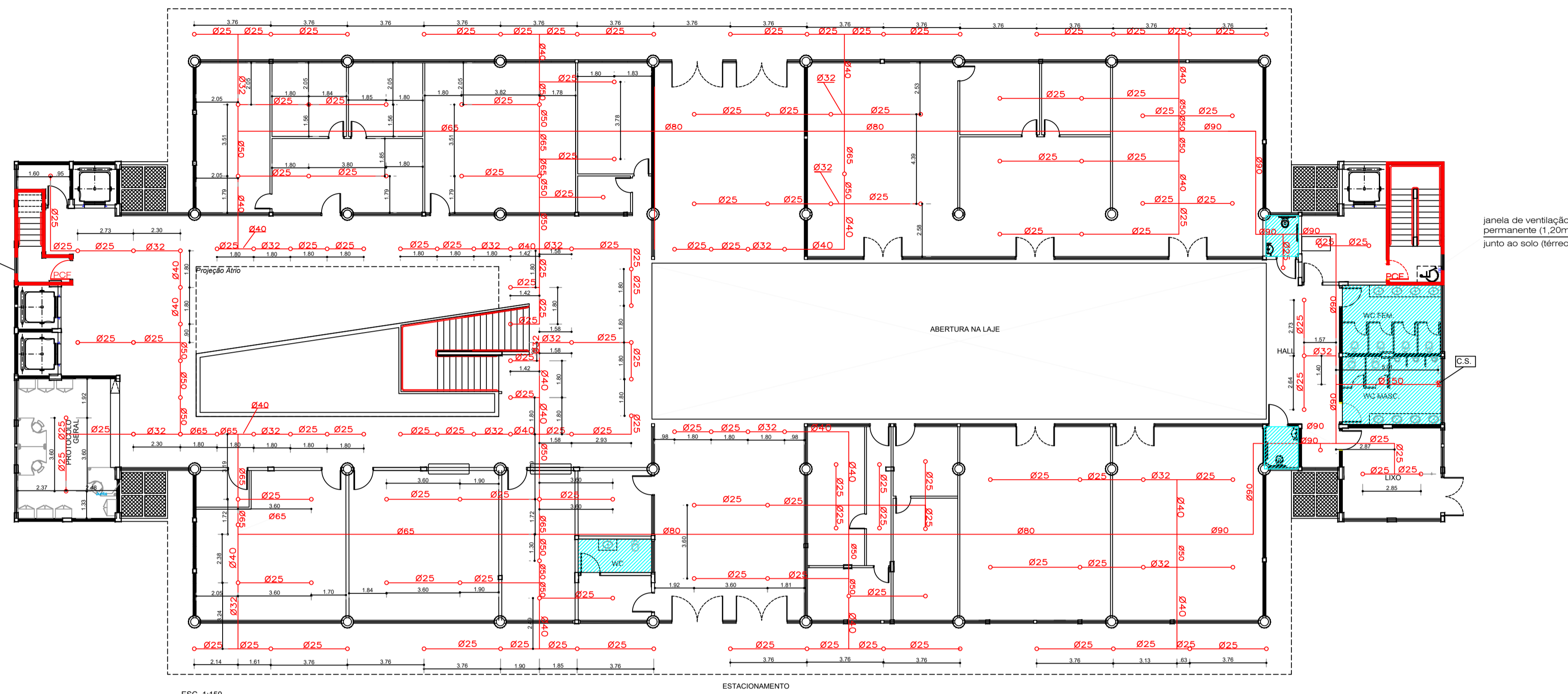
ESC. 1:150 PLANTA BAIXA - PAV. TÉRREO
