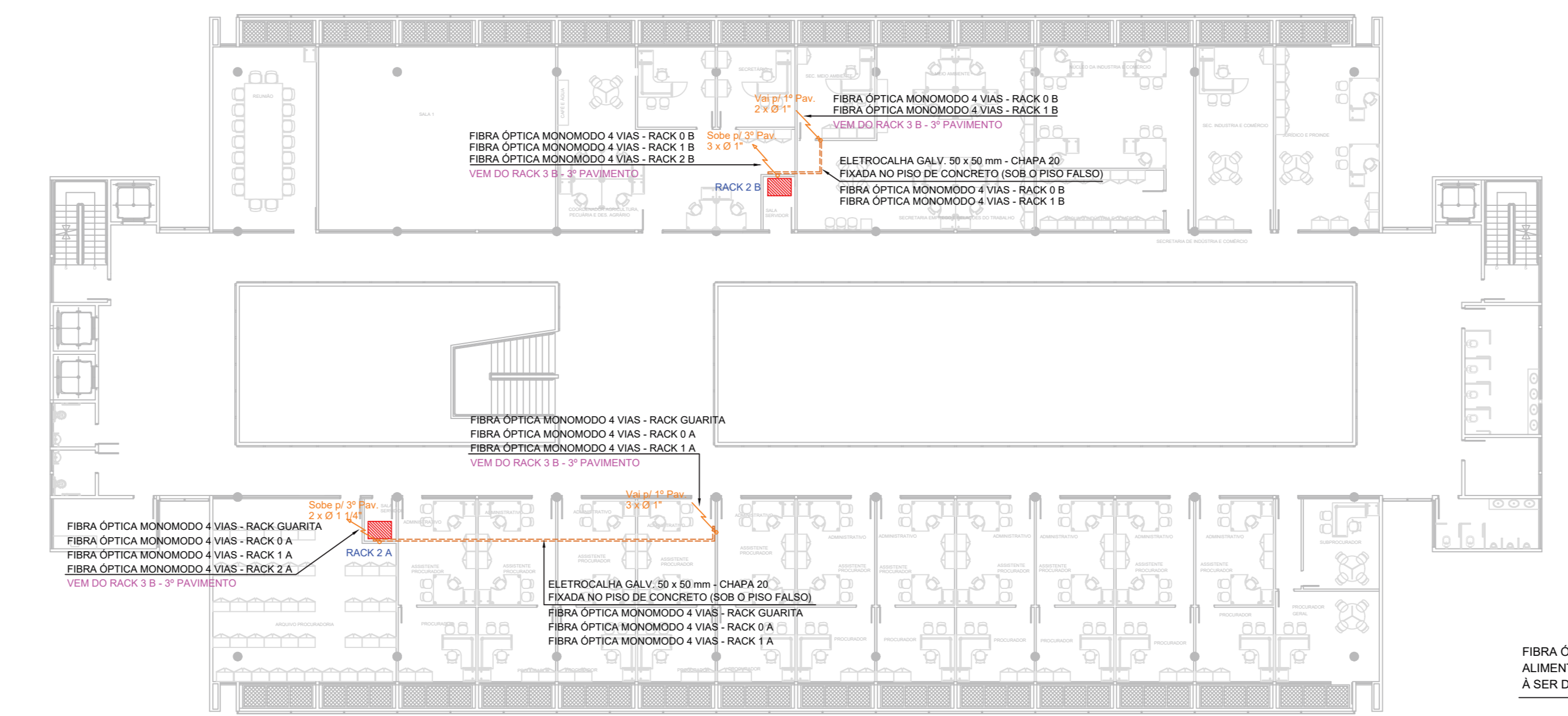
PLANTA BAIXA - 2º PAVIMENTO ESCALA 1:200
