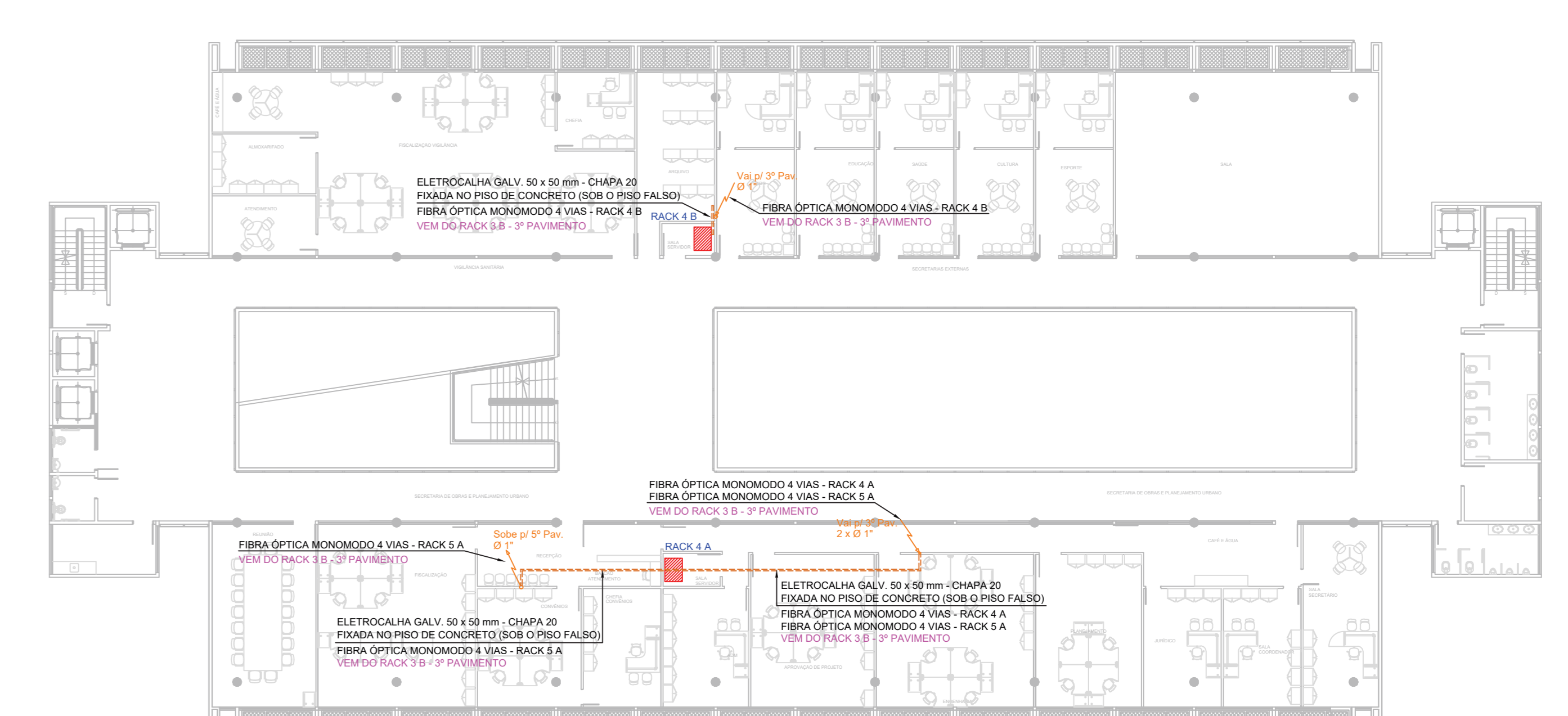
PLANTA BAIXA - 4º PAVIMENTO ESCALA 1:200
