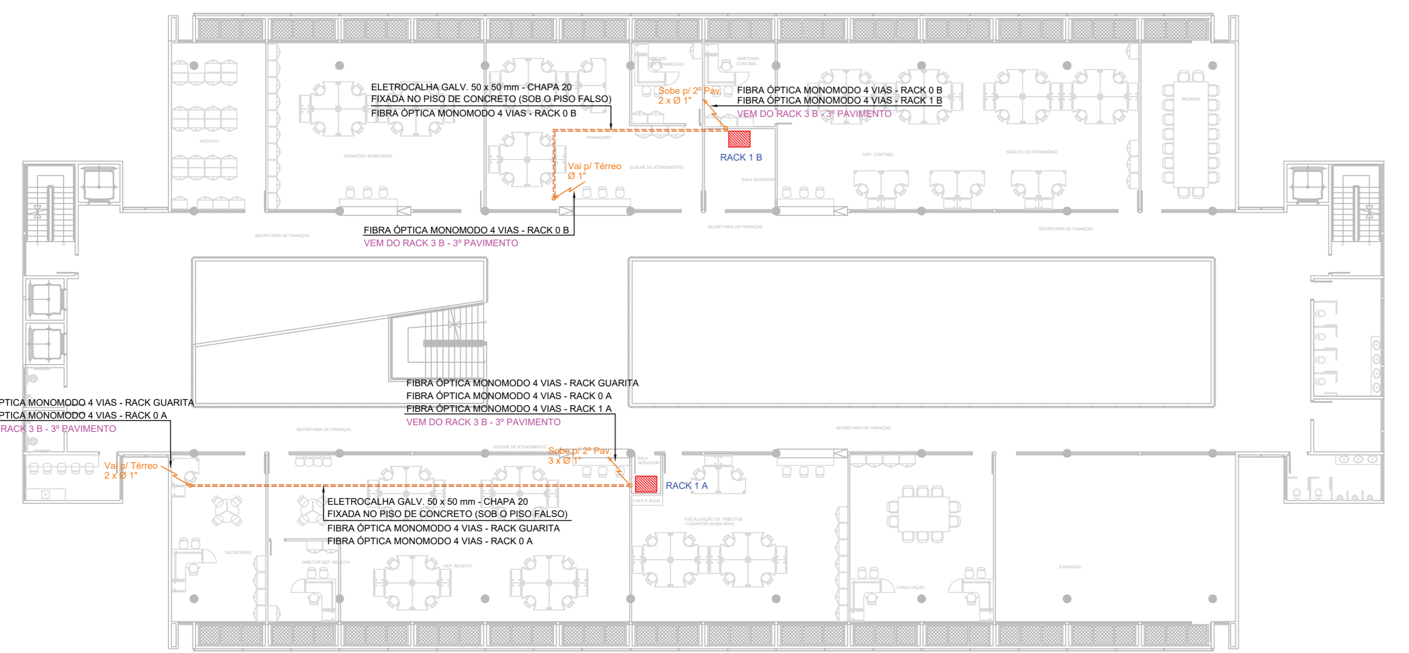
PLANTA BAIXA - 1º PAVIMENTO ESCALA 1:200
