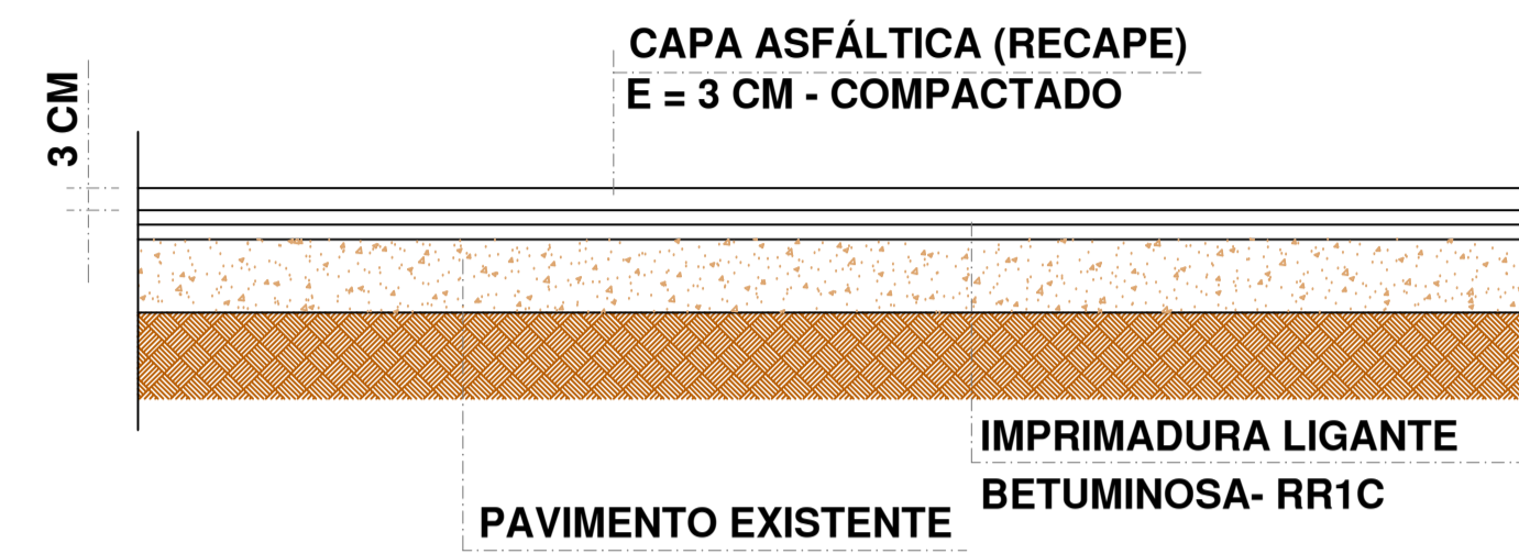
RECAPE DETALHE TÍPICO
