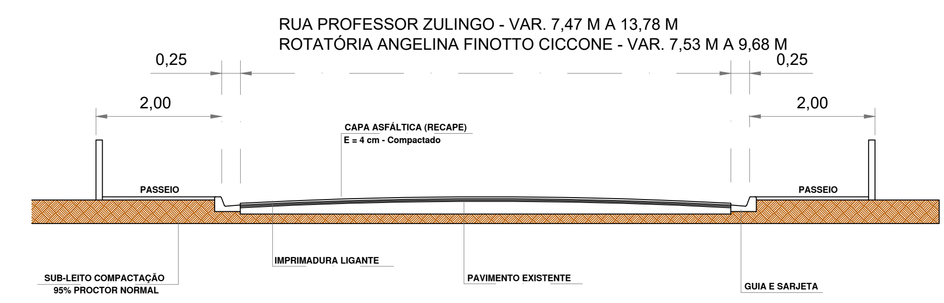
SEÇÃO TRANSVERSAL S/ ESCALA
