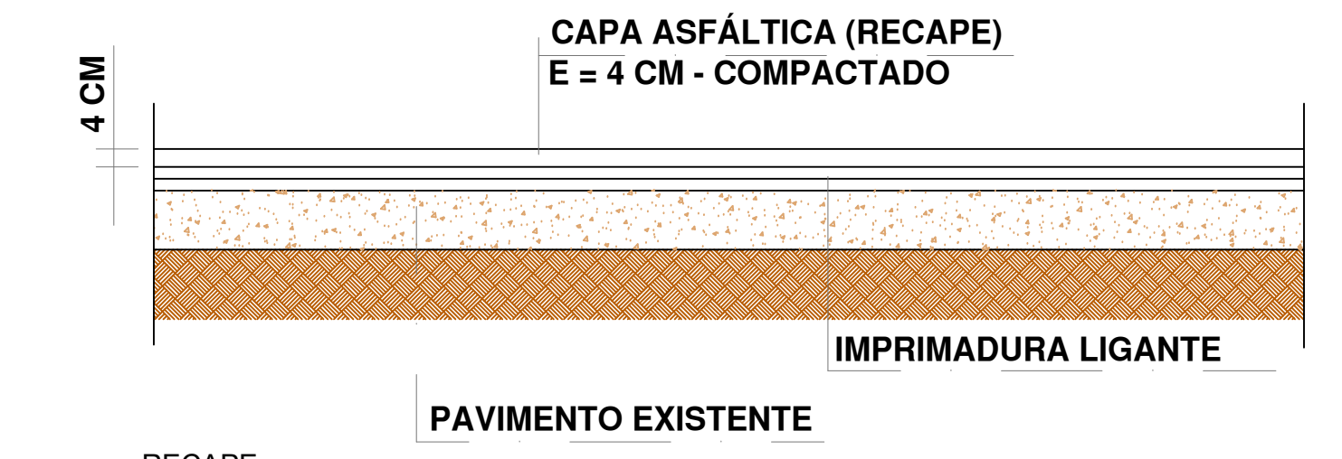
RECAPE DETALHE TÍPICO S/ ESCALA
