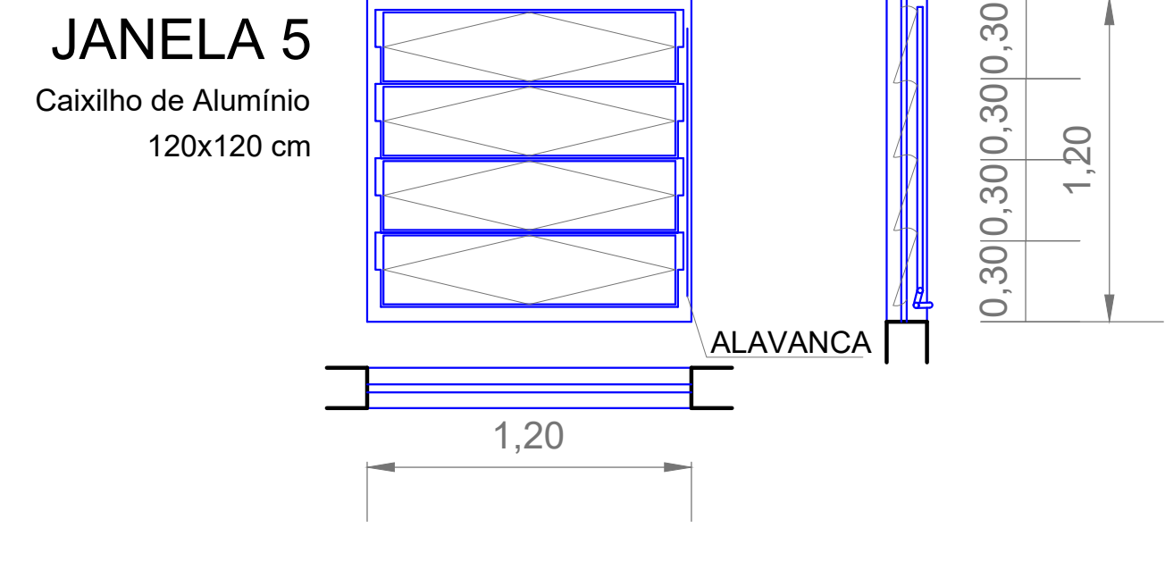
DETALHAMENTO DE ESQUADRIAS ESCALA 1:25
