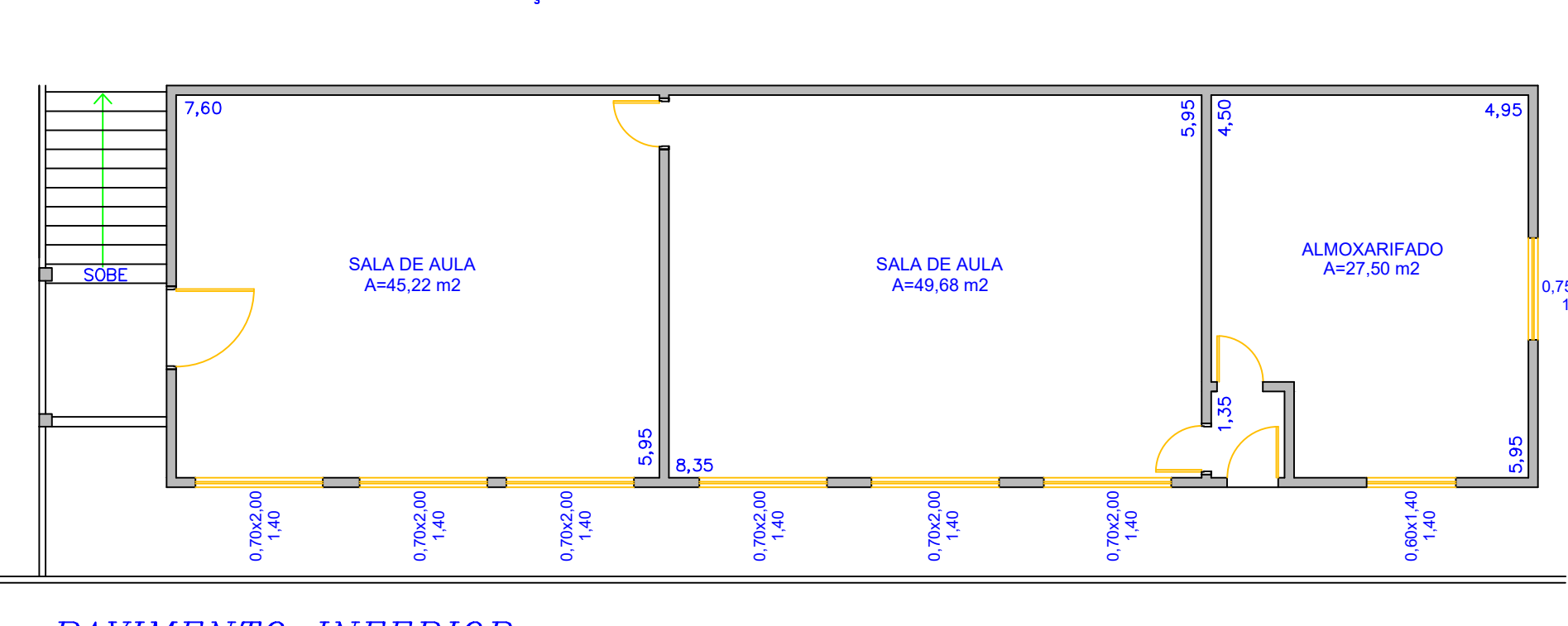
PAVIMENTO INTERIOR ESCALA 1:100
