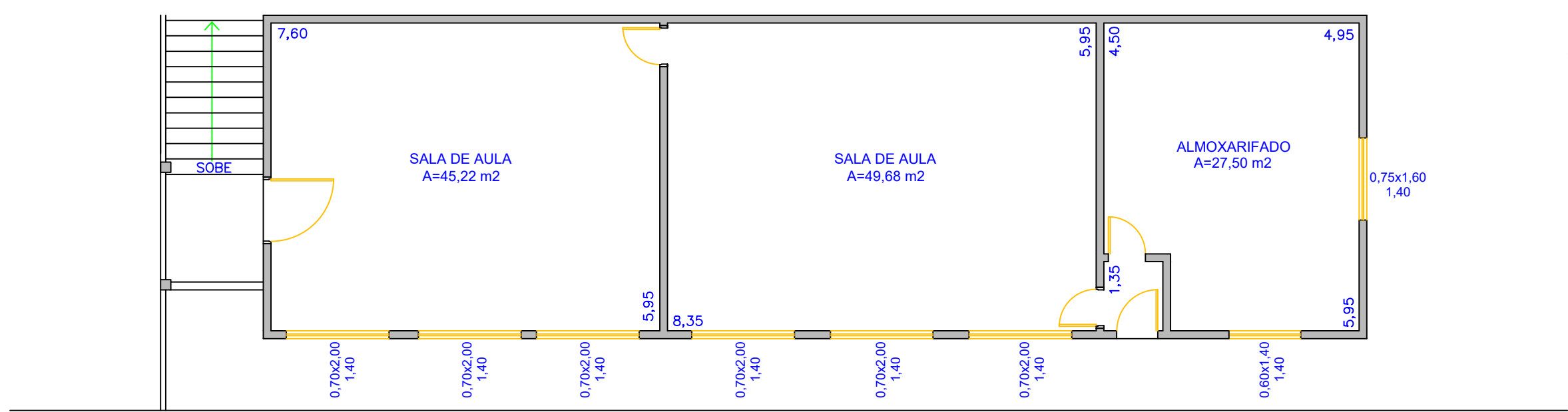
PAVIMENTO INTERIOR ESCALA 1:100
